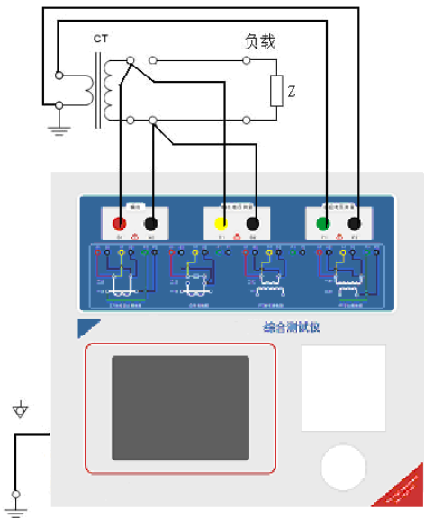
图 2.1 CT 直阻、励磁、变比试验接线方式
