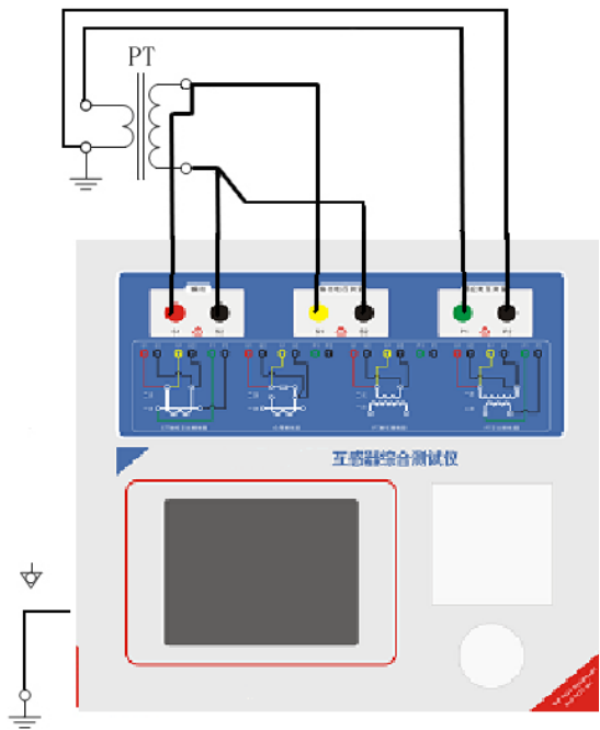
图 2.8 PT 变比、极性试验接线方式
