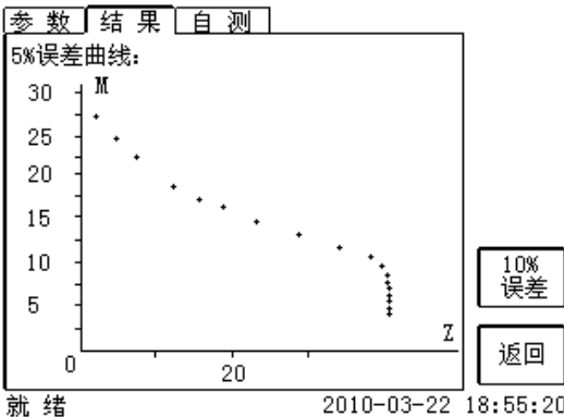
图 2.17 10%误差曲线界面
