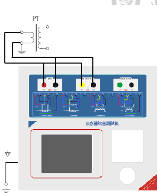
图 2.7 PT 直阻、励磁试验接线方式
