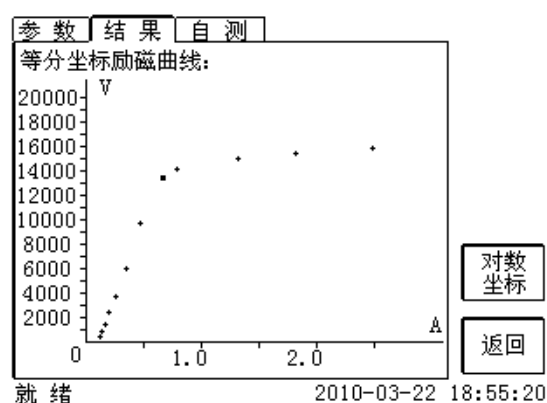
图 2.19 励磁曲线界面
